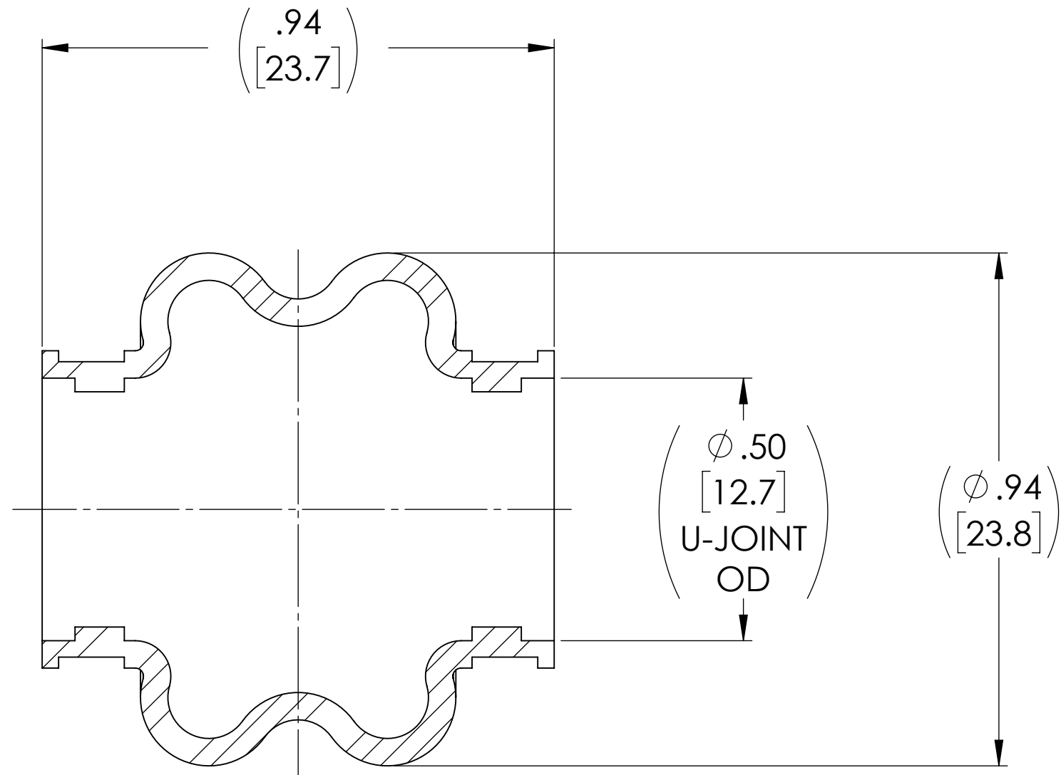
SECTION A-A
