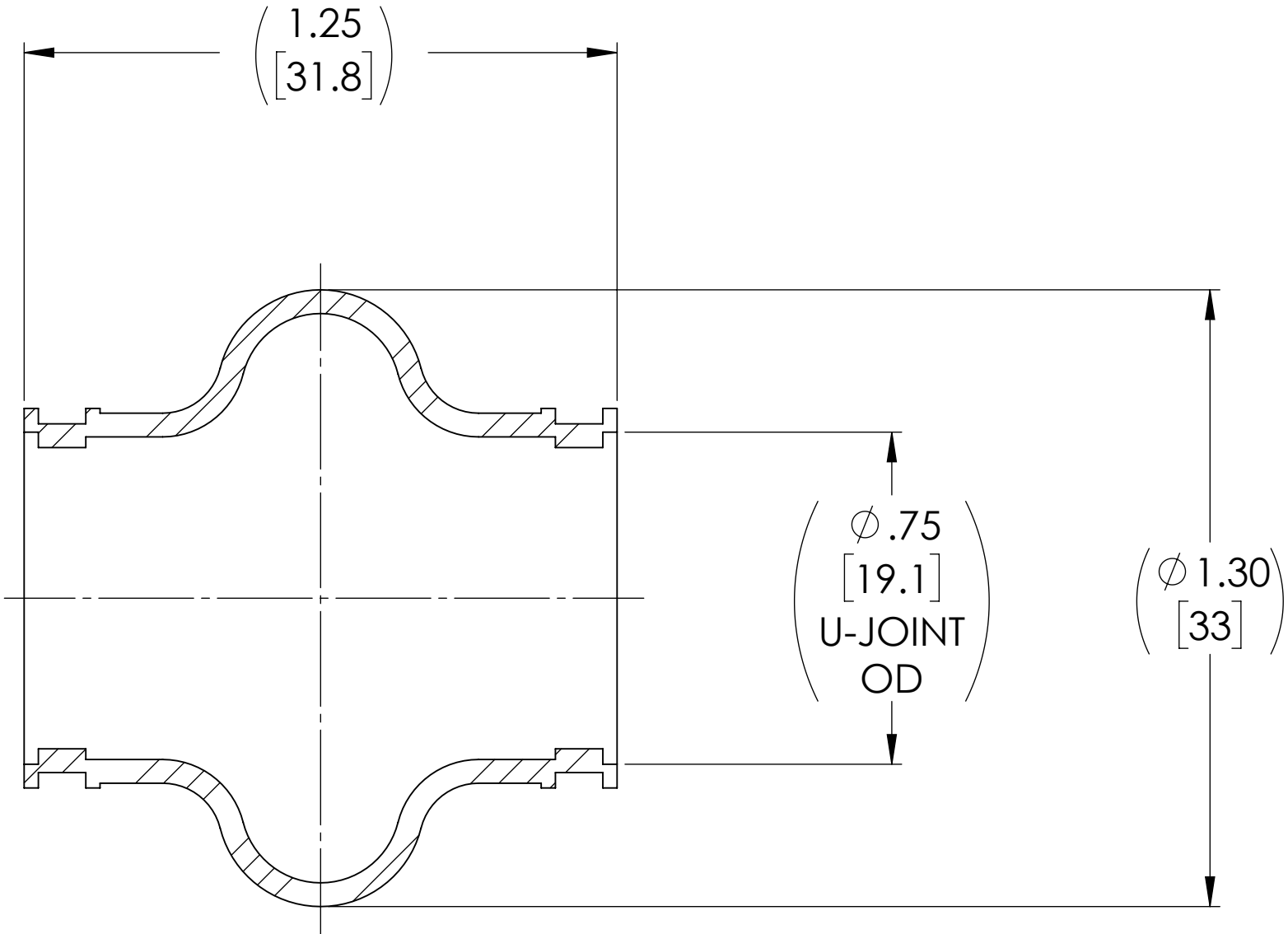
SECTION A-A
